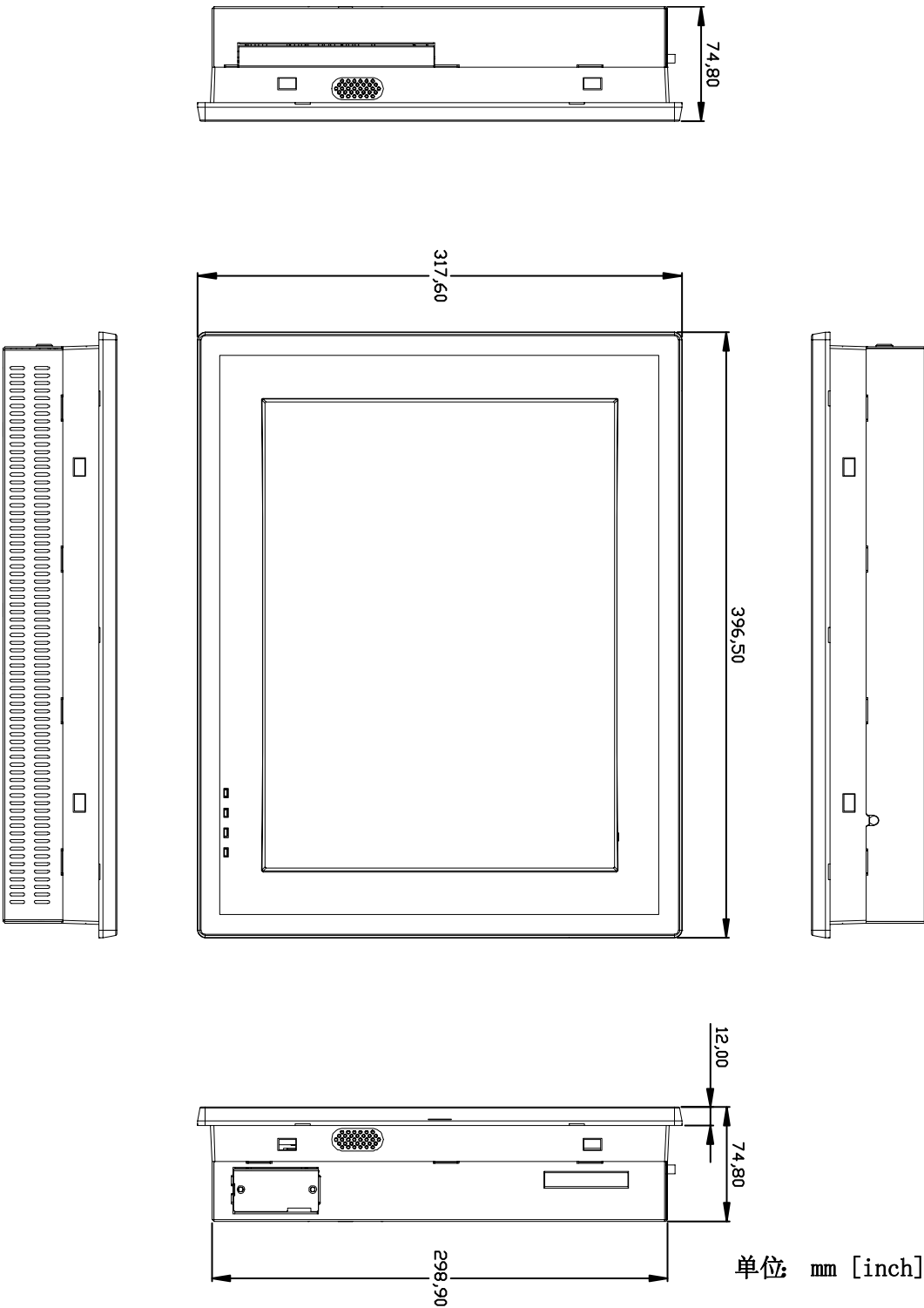
图 1.1: PPC-L157T 尺寸图
