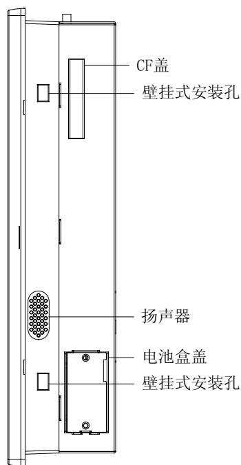
图 2.3: PPC-L157T 侧视图
